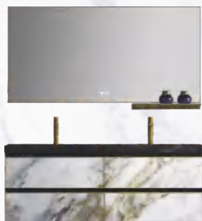
A-9004 主柜尺寸: 1400*550*550mm 智能镜尺寸: 1400*700mm 层架尺寸: 450*110mm 台面材质: 澳洲沙岩岩板台面 柜体材质: 多层生态板
